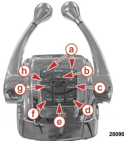
Elektronische Fernschaltung mit DTS Trackpad
