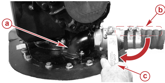
Typischer Seewasser-Einlasshahn – Backbordseite (Steuerbord ähnlich)
