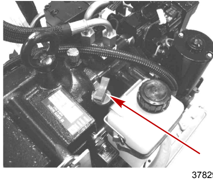
Getriebeölmesstab
